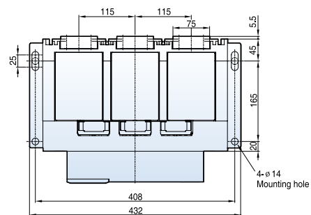
3P
