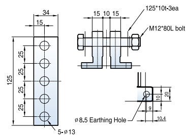
<Conductor>
