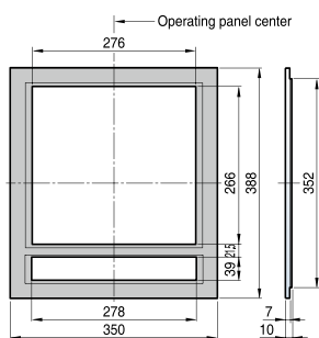
&lt;External size&gt;
