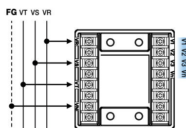
3P3W wiring
