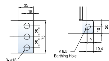
<Conductor>
