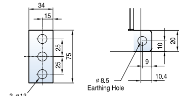
<Conductor>
