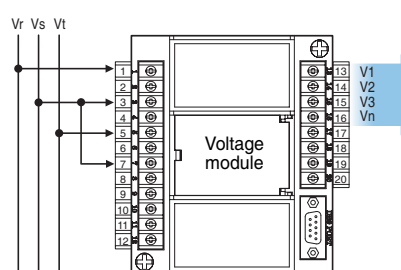
3P3W wiring
