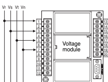
3P4W wiring
